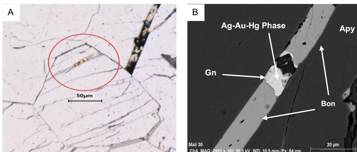
Abbildung 34: A: Ag-Au-Hg Phase zusammen mit Fahlerz (grau) in Arsenopyrit (weiß) (Probe „Mali“), B: Ag-Au-Hg Phase mit Bournonit und Galenit verwachsen in Arsenopyrit (REM-BSE, Probe „Mali“)
