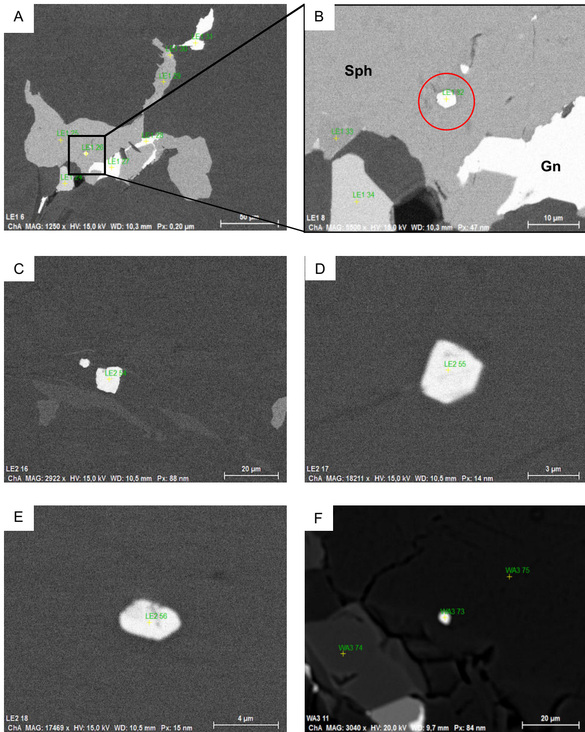
Abbildung 65: REM-BSE Bilder der Mikro-Uraninite Teil 1: A und B: Uraninit im Sphalerit (Probe LE1), C, D, E: Uraninite in den n. s. BM (Probe LE2), F: Uraninit in den n. s. BM (Probe WA3)
