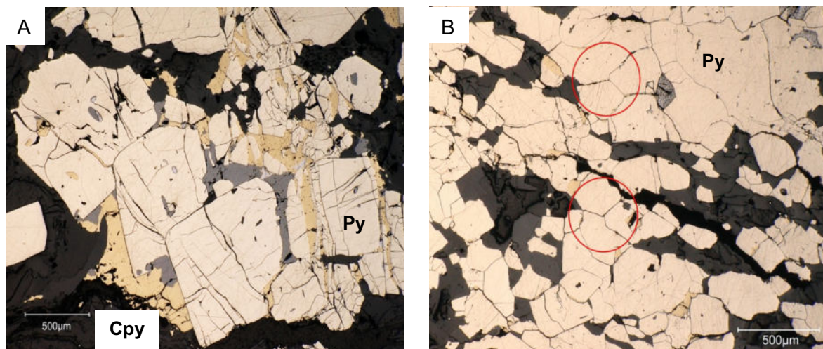
Abbildung 13: A: Kataklyse von Pyriten mit Chalkopyrit (gelb) als Rissfüller (LE2), B: Pyrit mit „triple-junction“-Verwachsungen (LE3)
