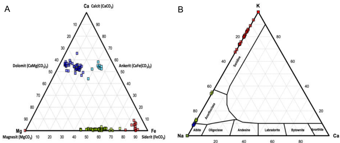
Abbildung 37: A: Vertreter der Karbonate im ternären Phasendiagramm (a.p.f.u.), B: Minerale der Feldspatgruppe im ternären Phasendiagramm (a.p.f.u.)
