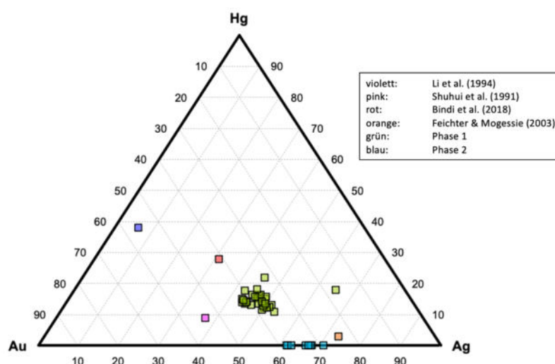
Abbildung 35: unterschiedliche Ag-Au-Hg Phasen im ternären Diagramm (in a.p.f.u. dargestellt)
