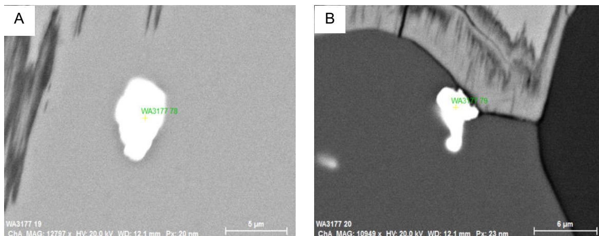
Abbildung 67: REM-BSE Bilder der Mikro-Uraninite Teil 3: A, B: Mikro-Uraninite in Magnetkies (A) und am Rand zu Magnetkies (B) (Probe WA3177)
