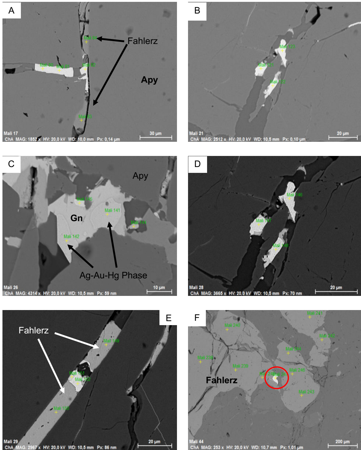
Abbildung 64: REM-BSE Bilder der Ag-Au-Hg Phasen Teil 2: A, B, D, E: Ag-Au-Hg Phasen zusammen mit Fahlerz in Arsenopyrit, C: Ag-Au-Hg Phase in Galenit, F: Ag-Au-Hg Phase in Fahlerz (alle Bilder aus Probe „Mali“)
