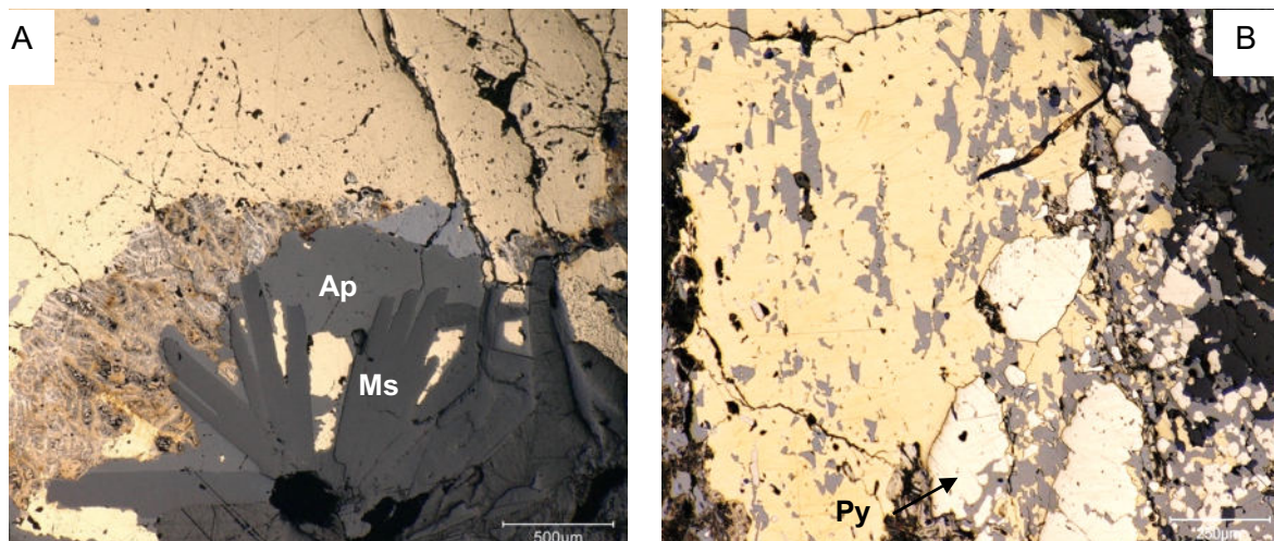
Abbildung 21: A: Chalkopyrit mit Pyrrhotin, Apatit und Muskovit ver wachsen (LE1), B: Kupferkies mit Sphalerit (grau) ver wachsen (WA3181)
