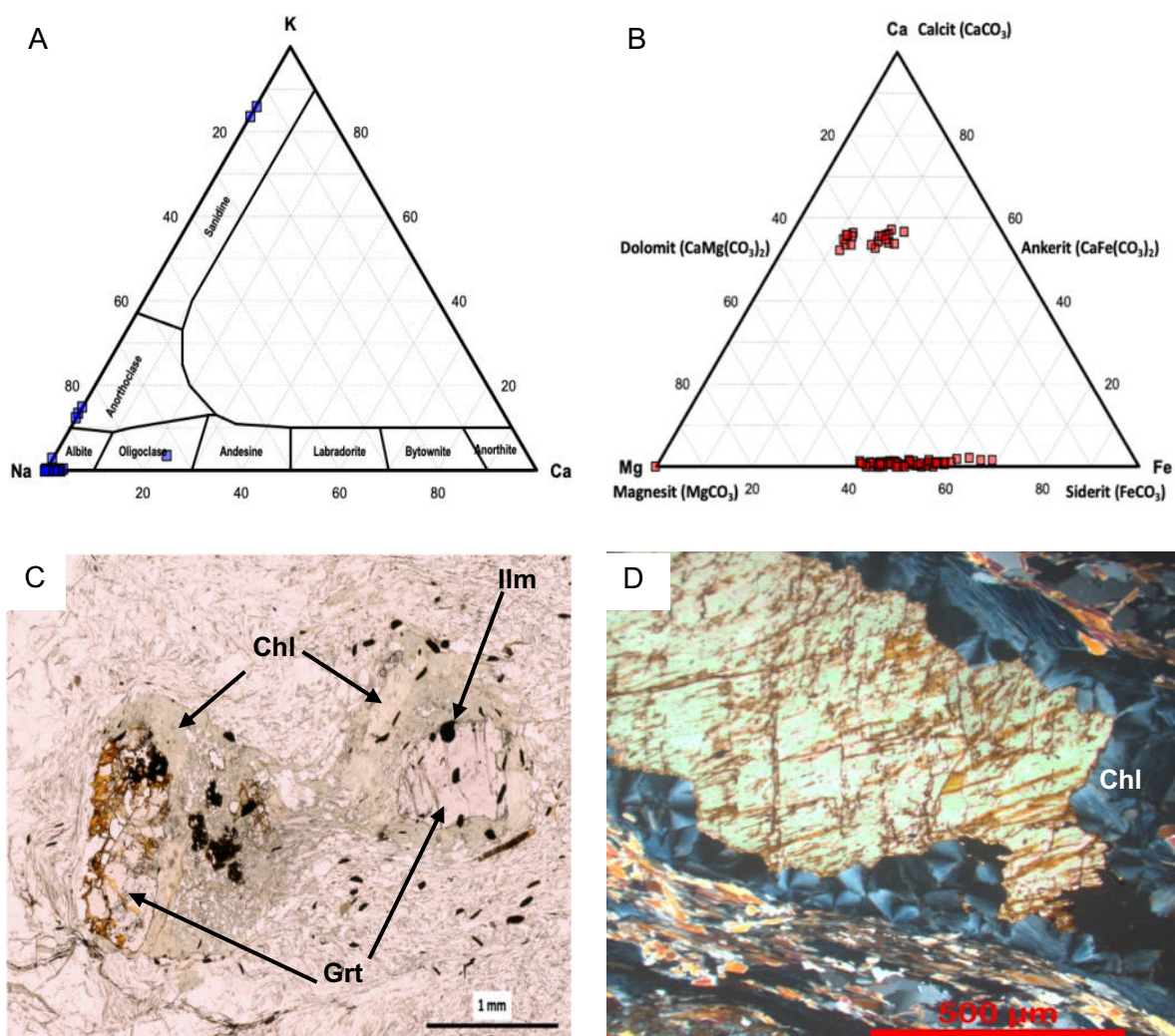
Abbildung 42: A: Vertreter der Feldspatgruppe im ternären-Phasendiagramm (a.p.f.u.), B: Vertreter der Karbonate im ternären Phasendiagramm (a.p.f.u.), C: Granatrelikte von Chlorit (grün) umhüllt mit Ilmenit Einschlüssen (schwarz) (//N, 19FM22), D: Karbonate mit charakteristischer Spaltbarkeit umrandet von Chlorit (+N, L01)
