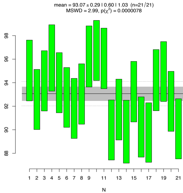
Abbildung 62: Berechnung des mittleren Bildungsalters der Mikro-Uraninite mittels IsoplotR-online
