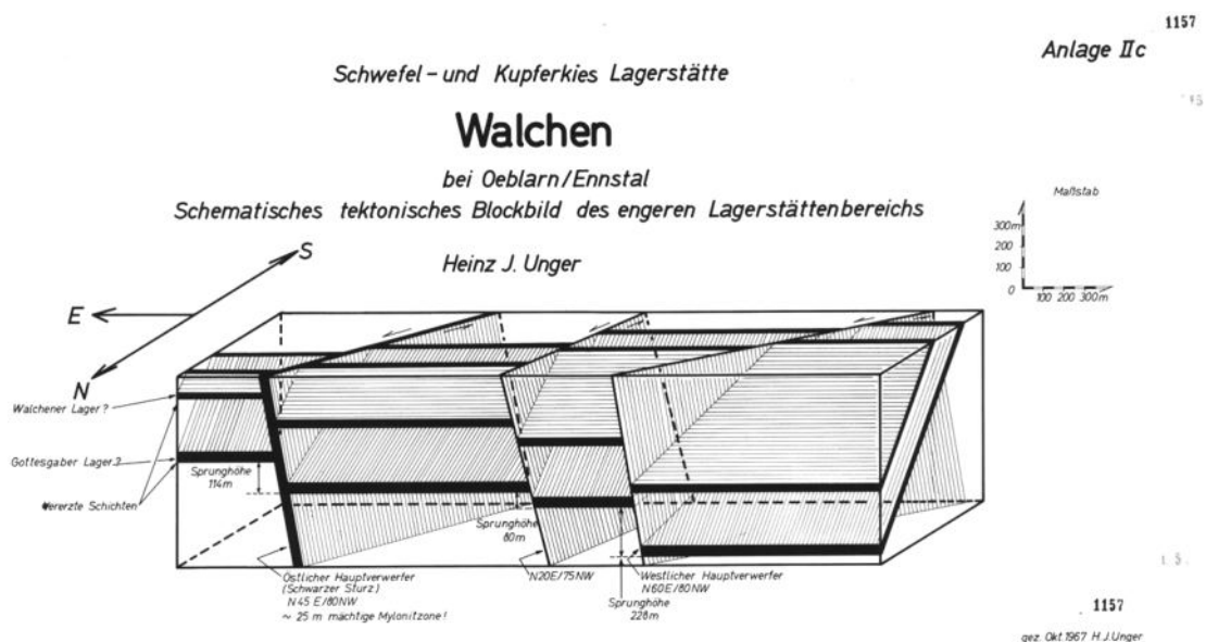
Abbildung 4: Tektonischer Bauplan der Lagerstätte (Unger, 1968)
