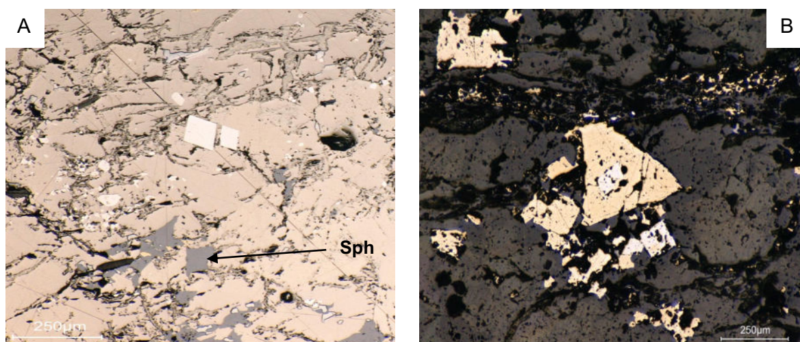
Abbildung 26: A: idiomorphe Arsenopyrit-Kristalle (weiß) ummantelt von Pyrrhotin (braun) (JA01), B: Arsenopyrit-Kristall (weiß) im Pyrit (gelblich)(19FM24)
