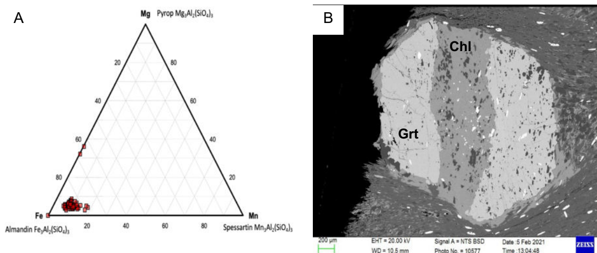
Abbildung 43: A: Vertreter der Granatgruppen Minerale im ternären Phasendiagramm (a.p.f.u.), B: Rotierter Granat mit Chlorit-Alteration (dunkelgrau) und Ilmenit-Einschlüssen (weiß) (REM-BSE, 19FM22)
