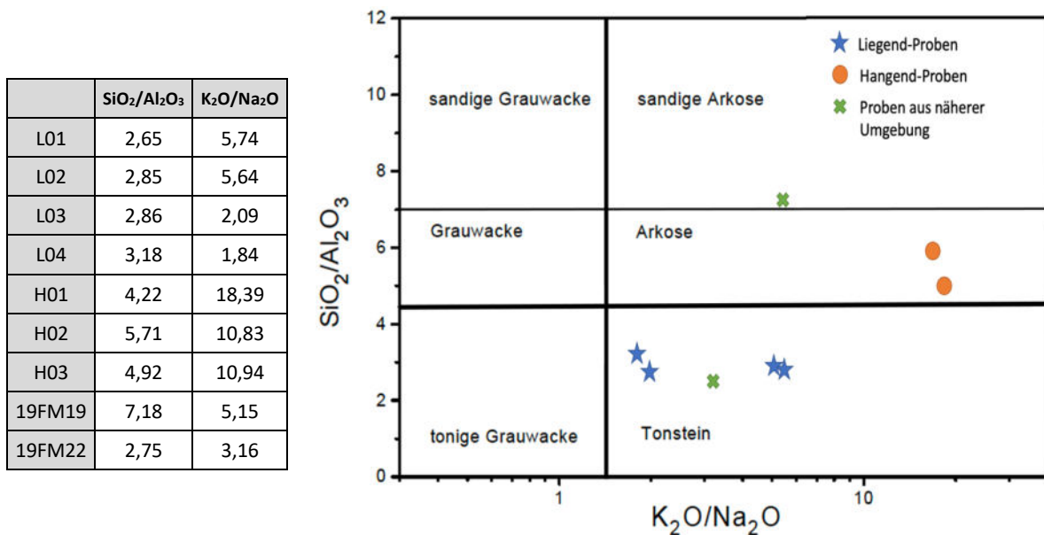
Abbildung 49: Unterteilung der Metasedimente mit dem Eduktdiagramm nach Wimmenauer (1984)
