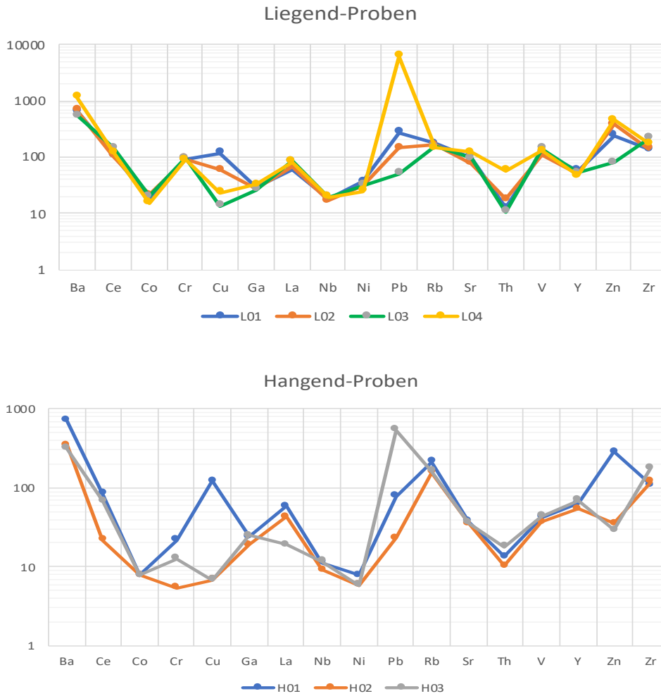
Abbildung 46: RFA Spurenelementverteilung in den Liegend- und Hangendproben aus dem Thaddäus-Stollen (in ppm)
