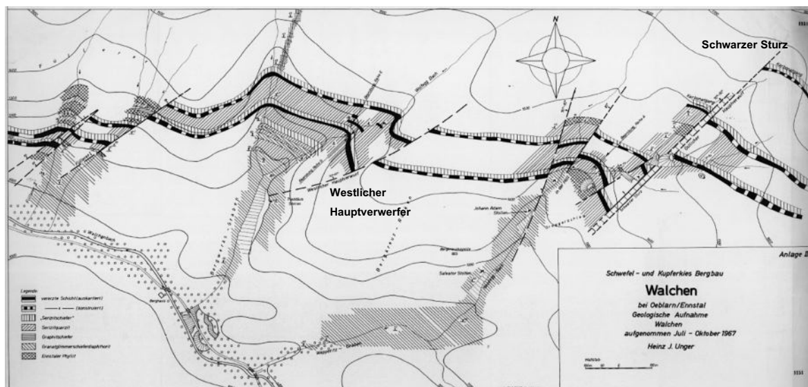
Abbildung 3: Kupferlagerstätte Walchen modifiziert aus Unger (1968)
