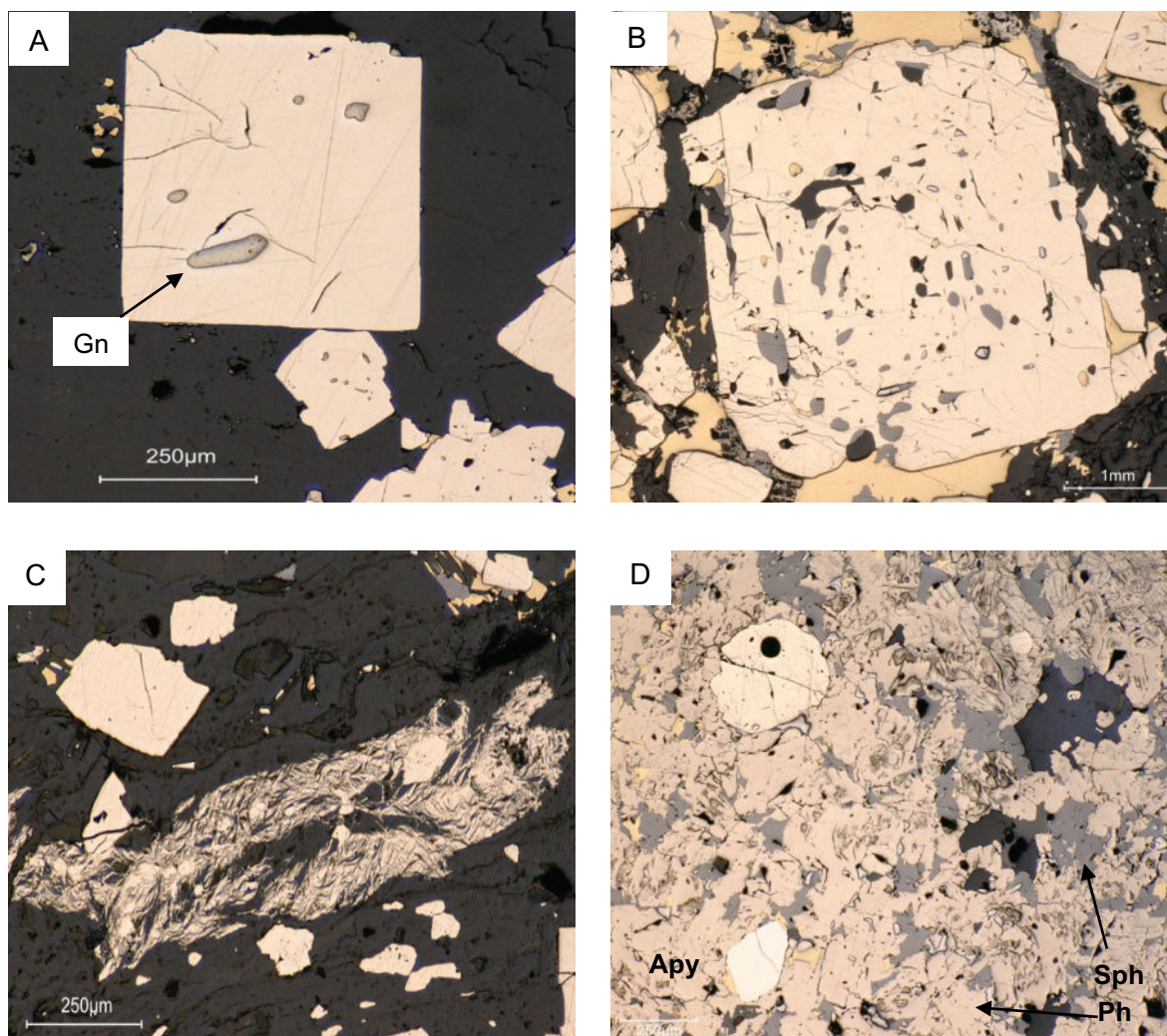
Abbildung 16: A: idiomorpher Pyrit (WA3185), B: Einschlüsse in Pyrit (WA3170), C: duktile Deformation (LE4), D: Pyrit umgeben von Pyrrhotin (WA2)
