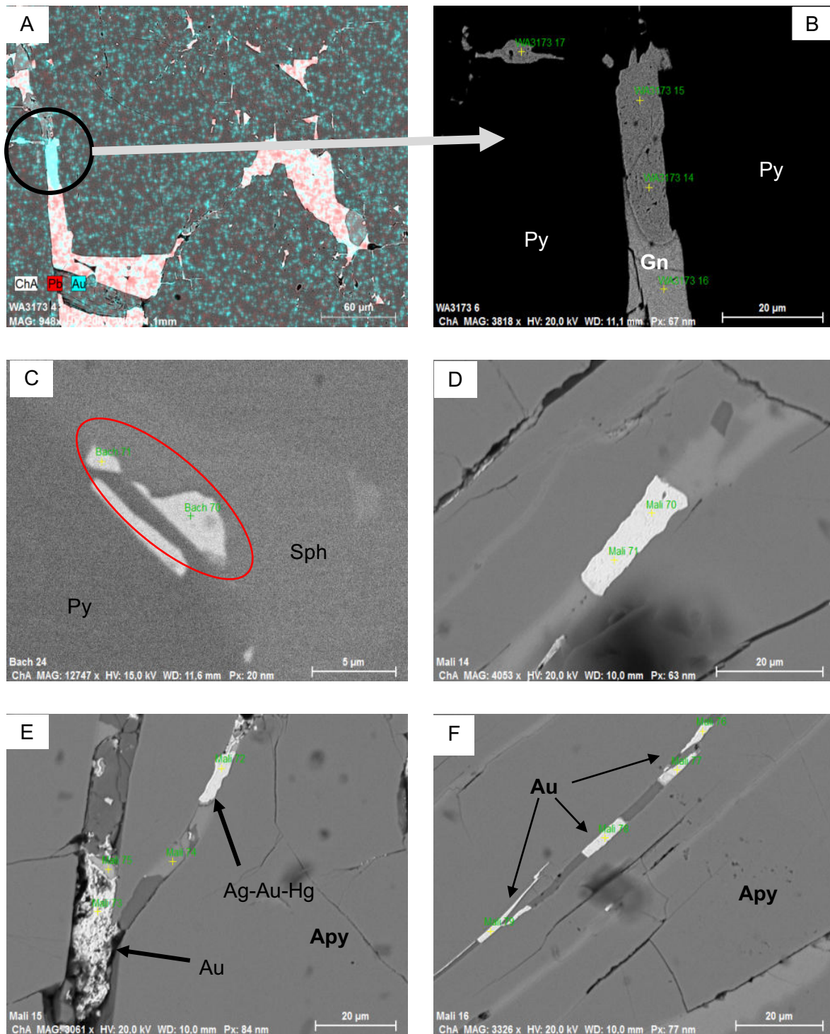
Abbildung 63: REM-BSE Bilder der Ag-Au-Hg Phasen Teil 1: Bild A (Element-mapping) und B (Probe WA3173), Ag-Au-Hg Phase in Pyrit, C: Ag-Au-Hg Phase zusammen mit Sphalerit in Pyrit (Probe Bach), D, E, F: Ag-Au-Hg Phase zusammen mit Fahlerzen in Rissen von Arsenopyrit (Probe „Mali“)
