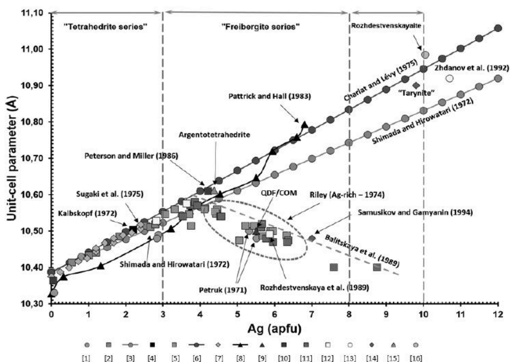
Abbildung 30: Beziehung zwischen Einheitszellenparameter und Ag-Gehalt (apfu) (Biagioni, et al., 2020)
