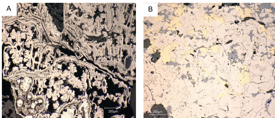
Abbildung 19: A: alterierter Magnetkies mit „birds-eye“ Struktur (Blei-Gang_1), B: Magnetkies verwachsen mit Chalkopyrit (gelb) und Sphalerit (grau) (WA3194)
