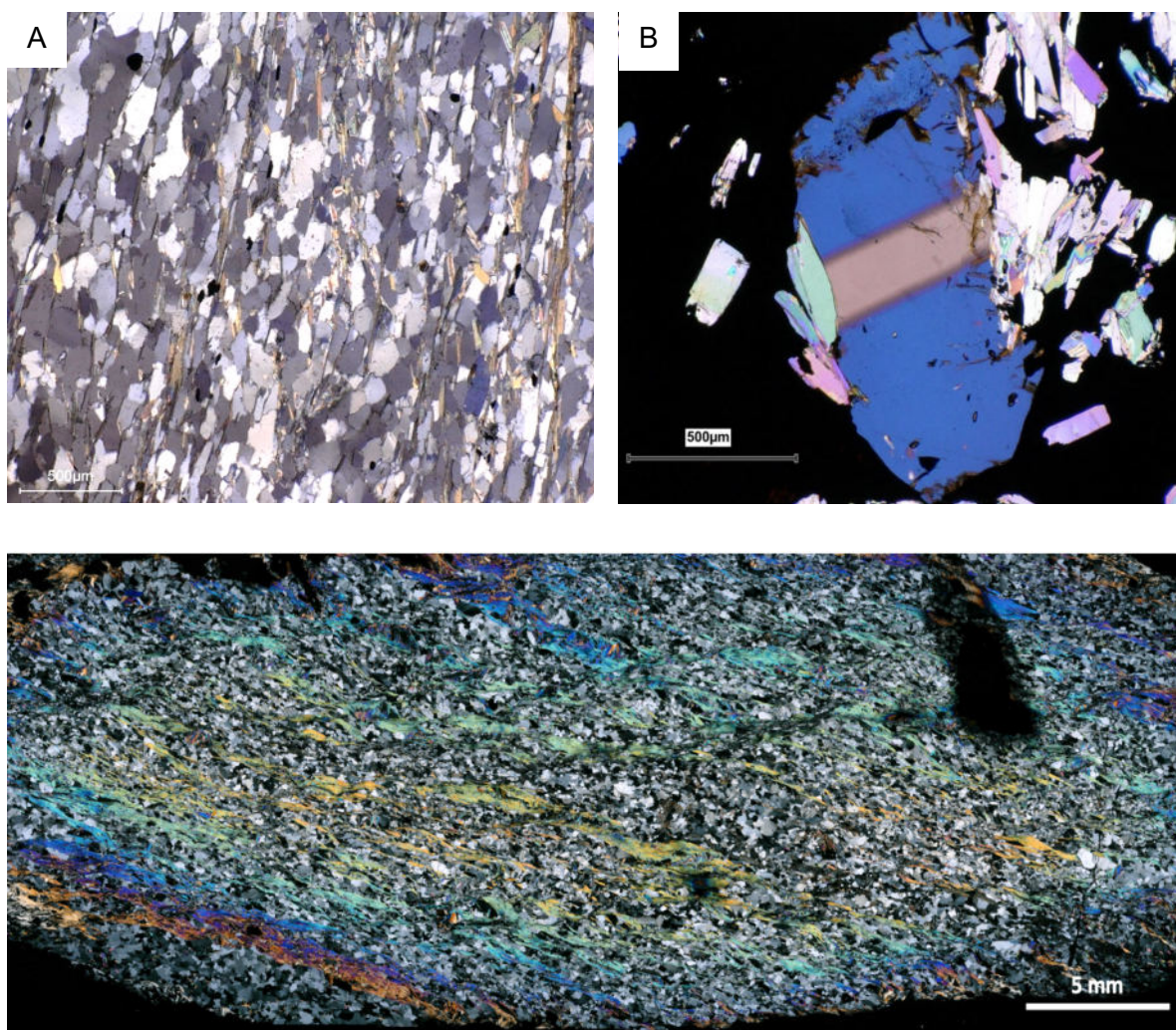
Abbildung 40: A: Einreglung von Quarzkristallen (+N, 19FM19), B: Böhmisches-Lamellen im Quarz umgeben von Muskovit (+ N, 19FM26), C: Panorama, farbig: Muskovit, schwarz/weiß: Quarz und Feldspatgruppen Minerale (+N, 19FM20)
