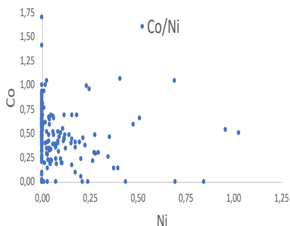
Abbildung 20: Boxplot Diagramm (Co, Ni) und Streudiagramm Co/Ni (m%)
