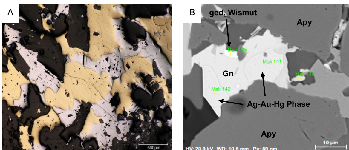
Abbildung 28: A: Galenit mit Dreiecks-Ausbrüchen verwachsen mit Kupferkies (gelb) (WA3180), B: Galenit mit Bi-Sb Phasen Einschluss verwachsen mit Ag-Au-Hg Phasen (REM-BSE, Probe „Mali“)
