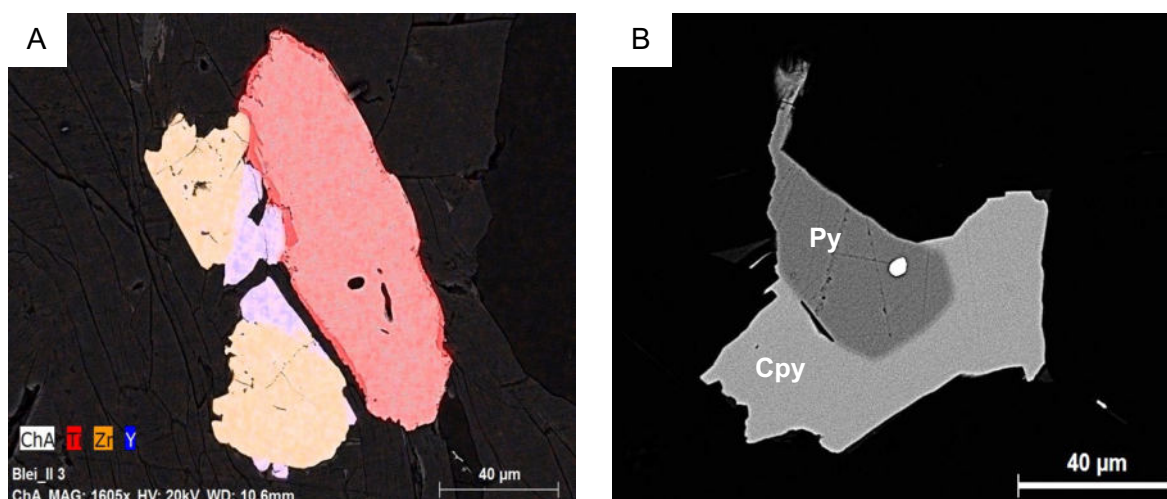
Abbildung 39: A: Verwachsung von Ilmenit (rot), Zirkon (orange) und Xenotim (blau) (Element Mapping, REM-BSE, Probe: Blei_2), B: Uraninit (weiß) Einschluss in Pyrit (dunkelgrau) (REM-BSE, Probe: WA3170)
