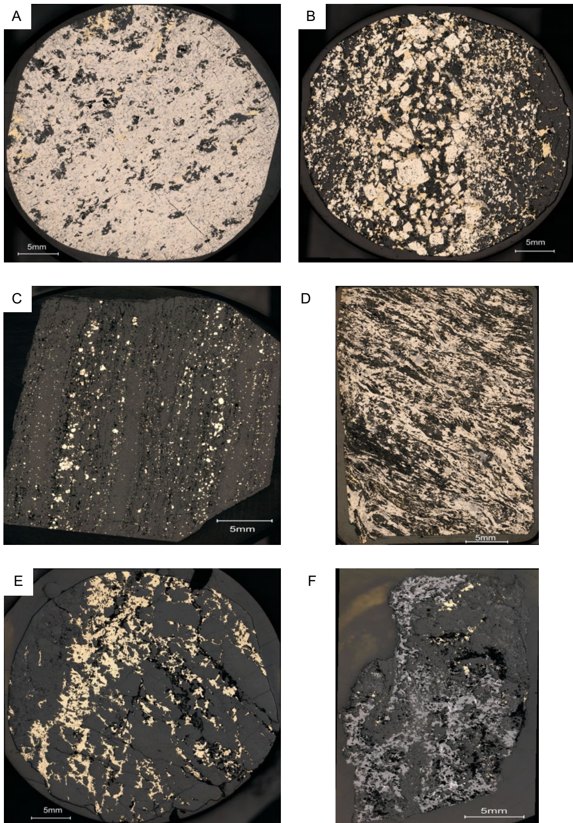
Abbildung 14: Unterschiedliche Erzgefüge A: Derberz (JA01), B: Py-IE_1 (WA3170) C: Py-IE_2 (FG01), D: Ph-IE (WA4), E: Cpy-IE (WA3196), F: Sph-IE (WA3187)
