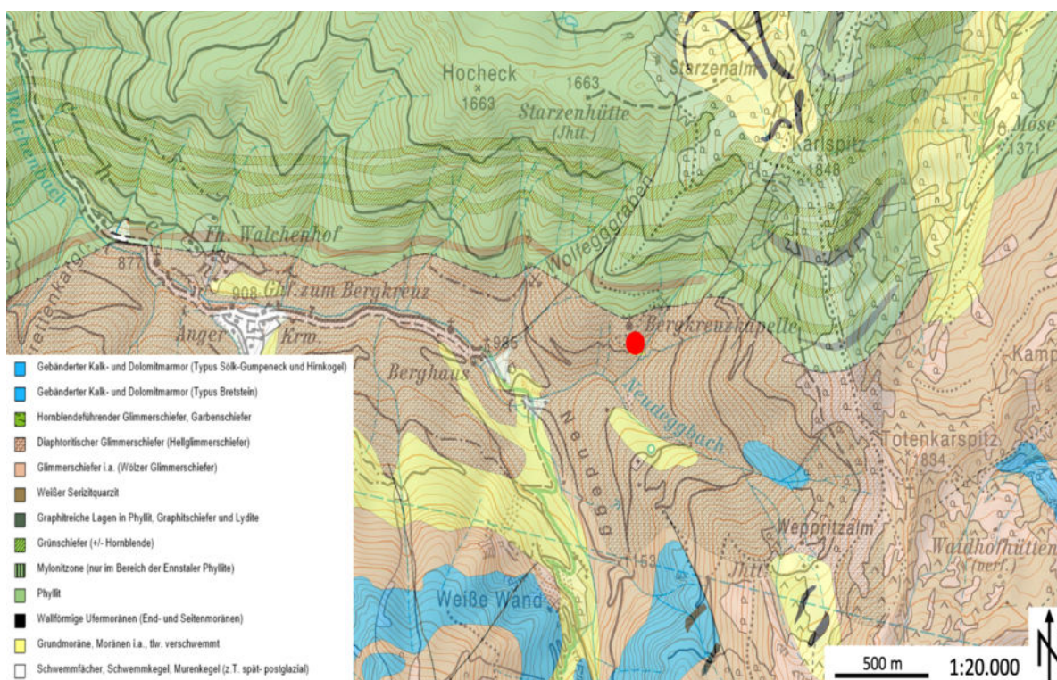
Abbildung 2: Geologischer Überblick Walchen, Lagerstätte (roter Punkt) (Quelle: GIS Steiermark)
