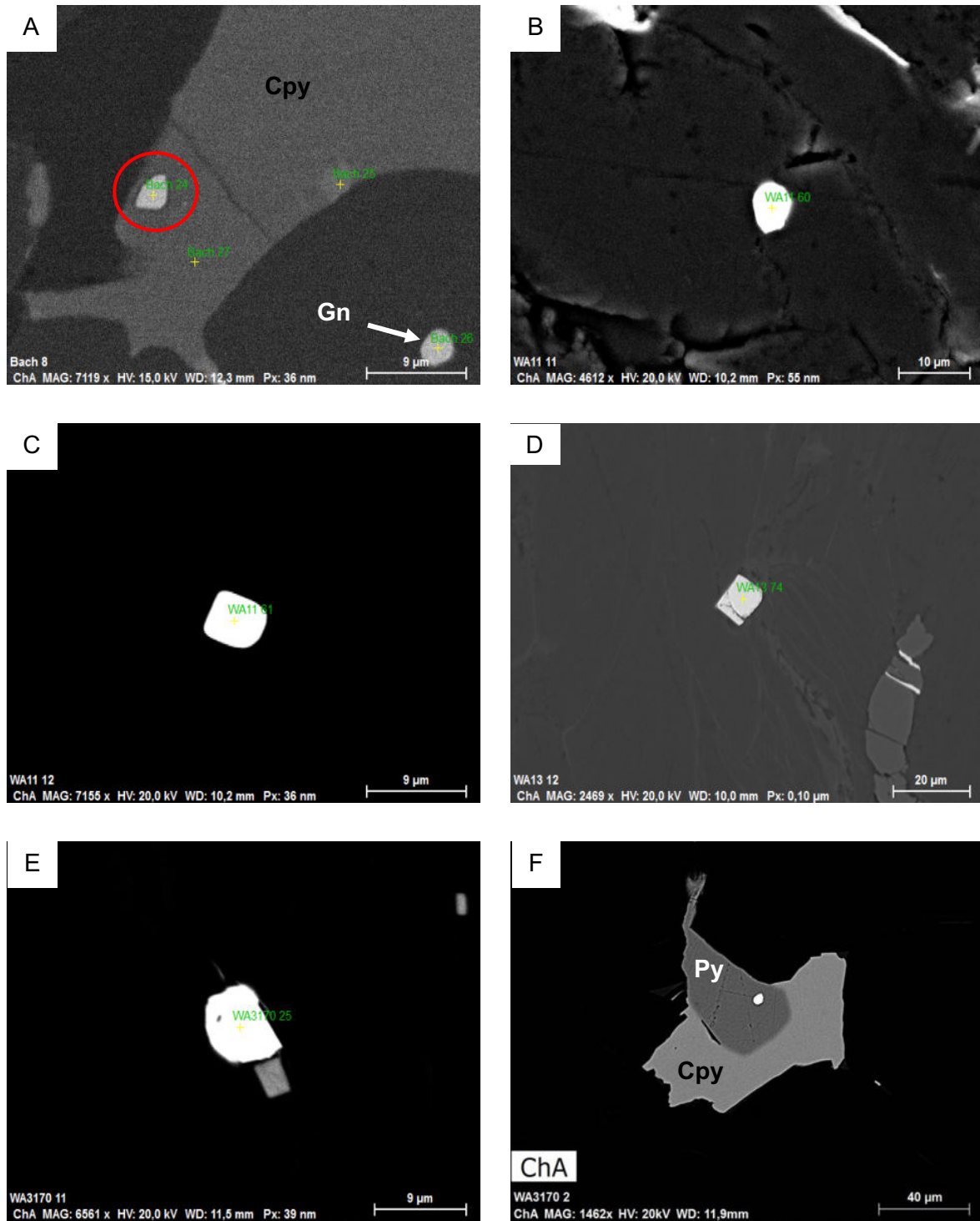
Abbildung 66: REM-BSE Bilder der Mikro-Uraninite Teil 2: A: Uraninit im Chalkopyrit (Probe Bach), B, C: Uraninite in den n. s. BM (Probe WA11), D: Uraninit in den n. s. BM (Probe WA13), E: Uraninit in den n. s. BM (Probe WA3170), F: Mikro-Uraninit in Pyrit (Probe WA3170)
