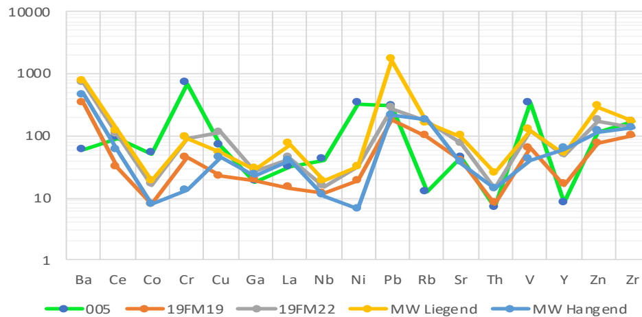
Abbildung 48: Vergleich von RFA-Spurenelementkonzentrationen in den Nebengesteinen (in ppm)
