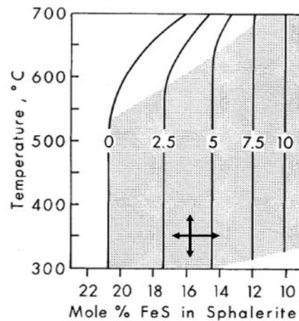
Abbildung 59: Graphische Darstellung des Sphalerit Bildungsdruckes nach Scott (1983)
