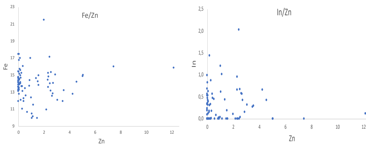
Abbildung 32: Streudiagramme Fe/Zn und In/Zn (m%)
