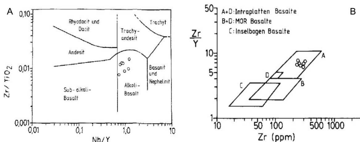
Abbildung 6: A: Diskriminierungsdiagramm für Metavulkanite aus Schlüter et al. (1984) B: Diskriminierungsdiagramm für tektonische Stellung aus Schlüter et al. (1984).
