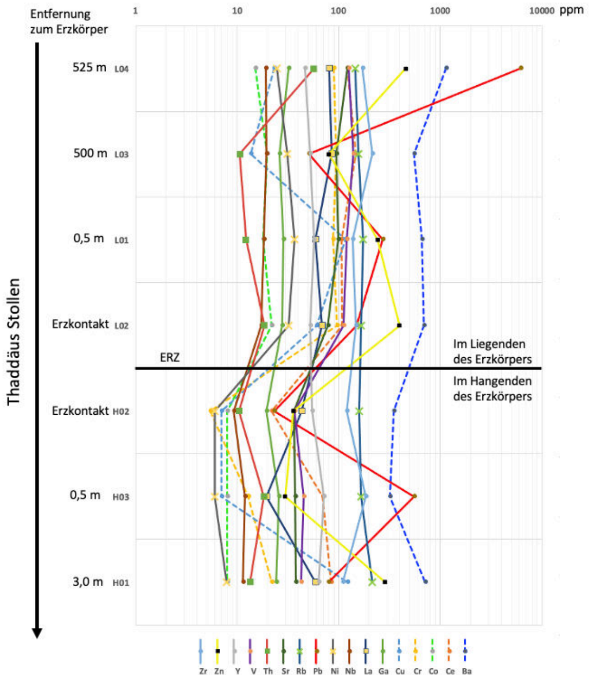
Abbildung 47: Veränderung der Spurenelementkonzentrationen (in ppm) im Stollenprofil
