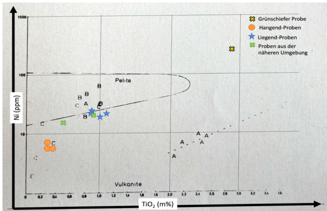
Abbildung 50: Ni-TiO 2 -Diagramm modifiziert nach Schlüter (1979), Kennzeichnung im Diagramm: A: Hornblendenschiefer, Grünschiefer und Biotitschiefer von dicht oberhalb der Vererzung, B: Serizitphyllite, Serizitquarzite und Granatglimmerschiefer aus der direkten Umgebung der Vererzung (Hangendes und Liegendes), C: Serizitphyllite und Serizitquarzite aus den vererzten Bereichen
