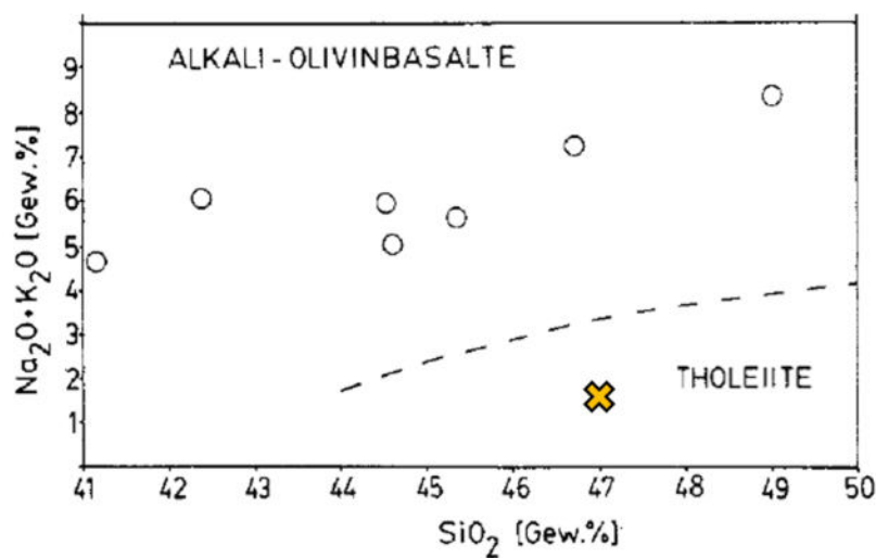
Abbildung 52: Diskriminierungsdiagramm für Basalte nach Schlüter et al. (1984), Oranges X: Grünschieferprobe (005), weiße Kreise: Grünschieferproben aus der Lagerstättenumgebung von Schlüter (1979)
