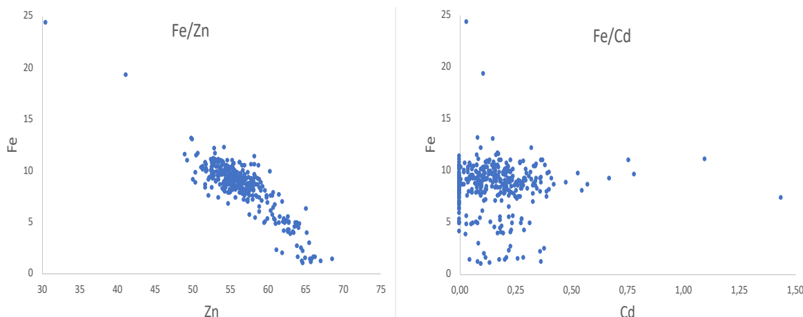
Abbildung 25: Streudiagramme Fe/Zn und Fe/Cd (m%)
