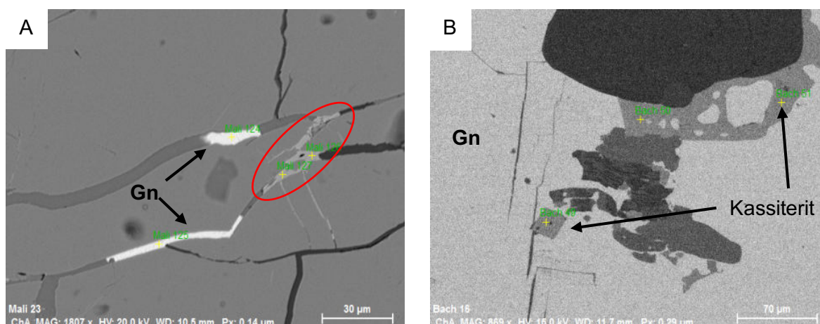
Abbildung 38: A: Kassiterit in Rissen von Arsenopyrit (Probe „Mali“), B: idiomorpher Kassiterit-Kristall in Galenit (links), xenomorpher Kassiterit mit Galenit Einschlüssen (Probe Bach)
